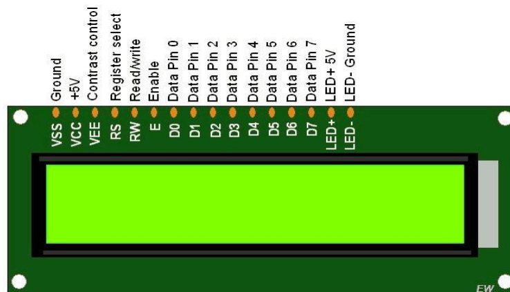
Fig. 2.7 16×2 LCD Display
